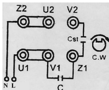
Rechtslauf/Rotation right
