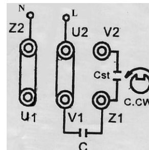
Linkslauf/Rotation left
